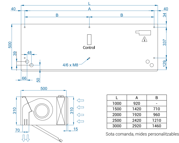
Instal·lació horitzontal
